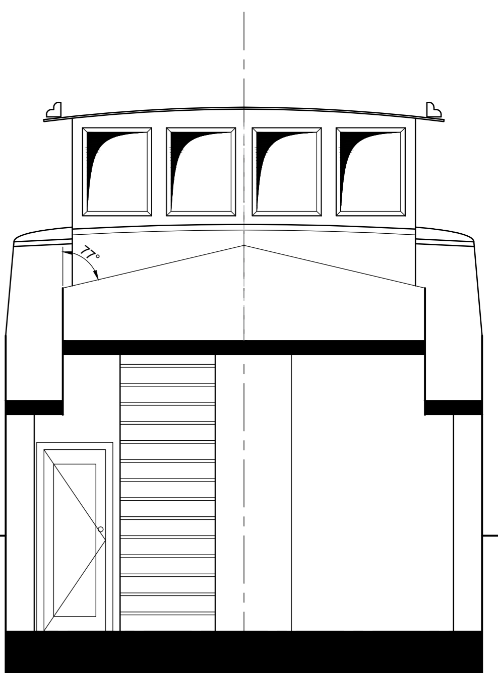
Doorsnede A-A Schaal: 1:40
